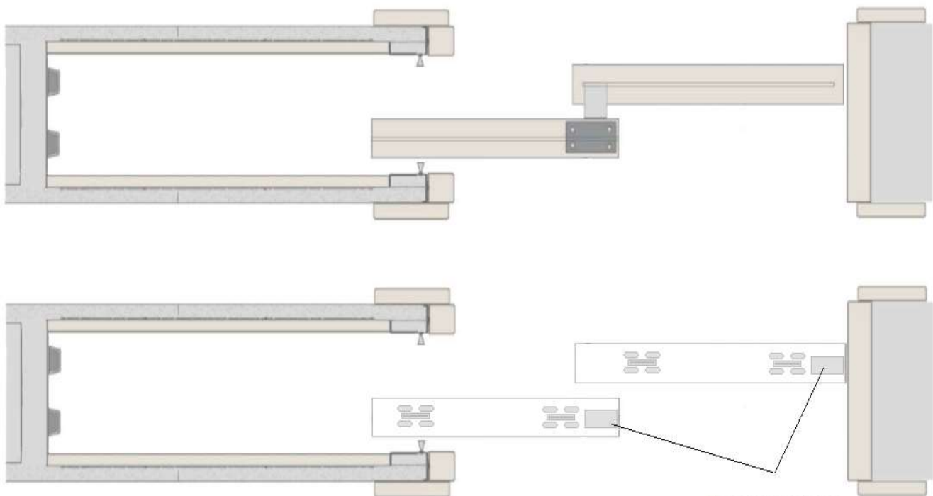
Door stooper
